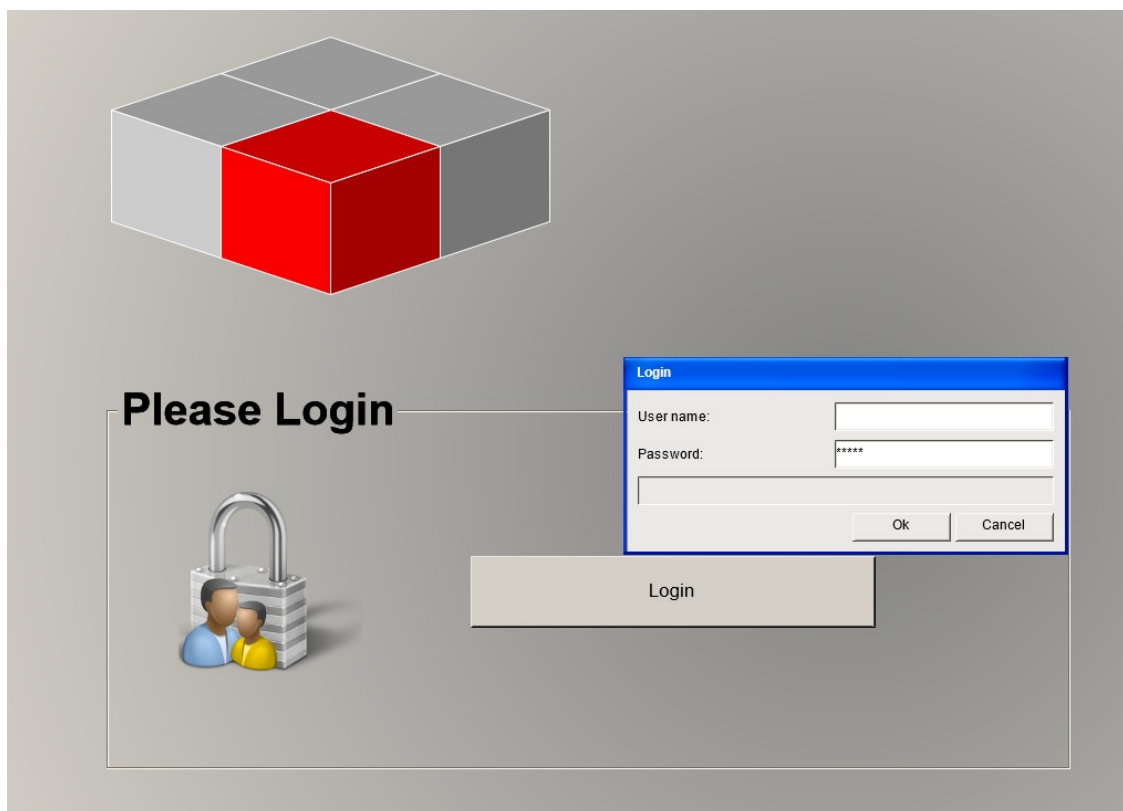
Login dialog
